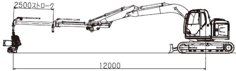
最長作業範囲
